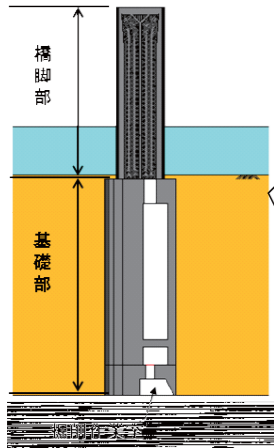
ニューマチックケーソン工法の概念図
